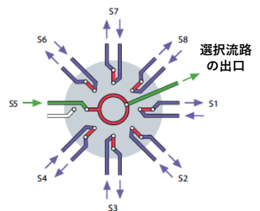
SF型の流路構成図
