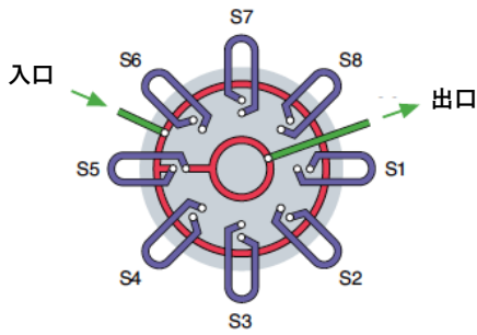
ST型の流路構成図
