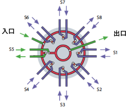
STF型の流路構成図
