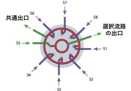
SC型の流路構成図
