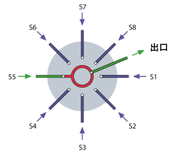
SD型の流路構成図
